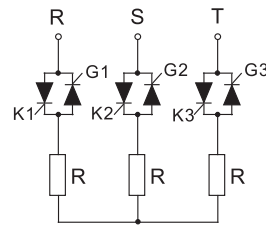
三相全控模塊
