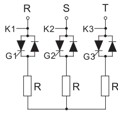
三相半控模塊
