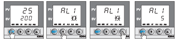
按下 SET 鍵切換至AL1 按下 ← 鍵切換到第一位數字 按下 ↑ 鍵增加警報設定值 按下 SET 鍵寫入警報設定值
