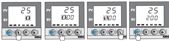
按下 ← 鍵SV數字開始閃動 按下 ← 鍵切換到第三位數字 按下 ↑ 鍵增加設定值 按下 SET 鍵寫入設定值
