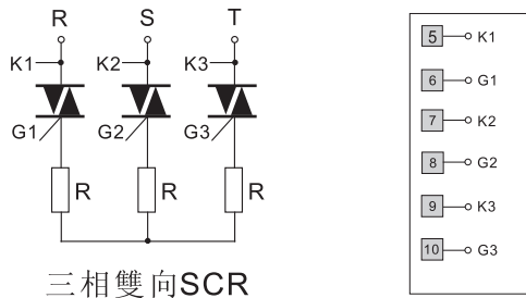
三相雙向SCR
