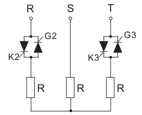
兩相全控模塊
