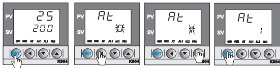
按下 SET 鍵切換至AT 按下 ← 鍵SV數字開始閃動 按下 ↑ 鍵設定成1 按下 SET 鍵後啓動Auto Tuning (AT燈亮)
