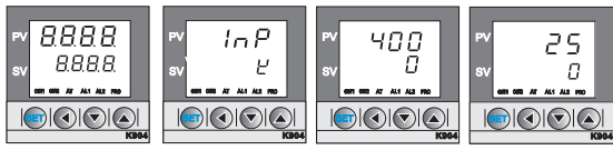
點亮所有LED及7段顯示器 顯示輸入感測器類型(K) 顯示上下限範圍(0~400) 開始使用
